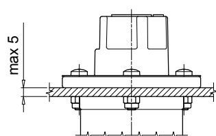
Montaggio esterno
