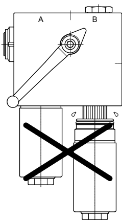
LATO ERRATO
